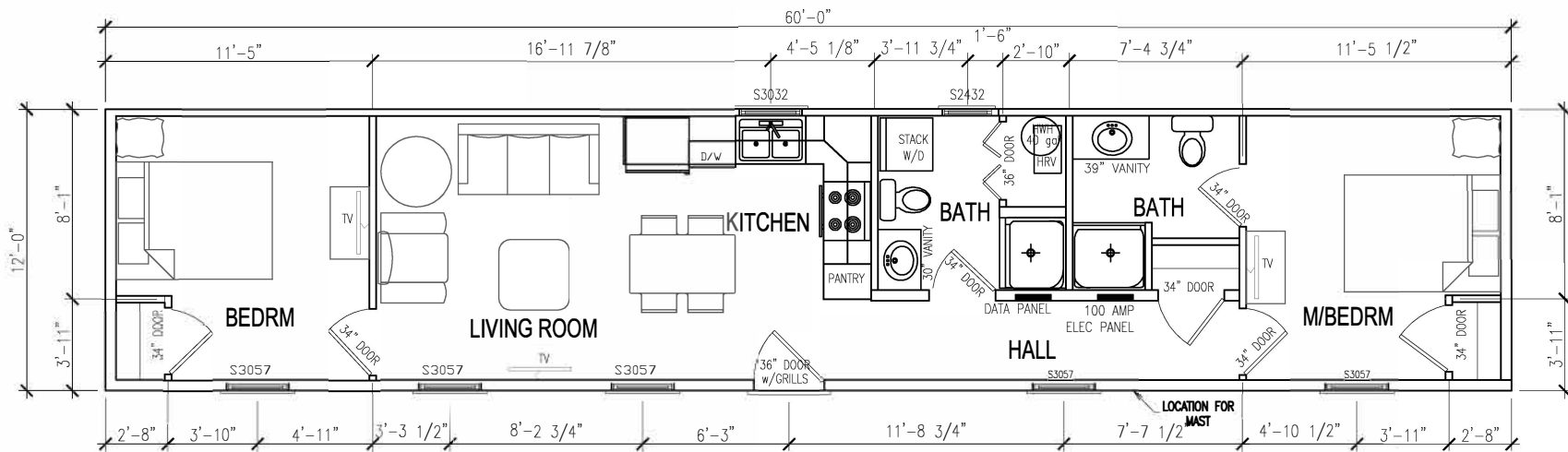
FLOOR PLAN SCALE: 1/8" = 1'-0"
